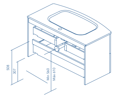
ROUND Fondo de tubería 7cm.
