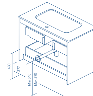
EASY Fondo de tubería 7cm.
