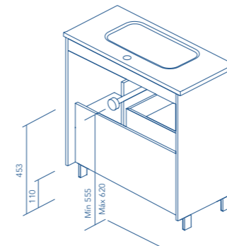
CONFORT Fondo de tubería 9cm.
