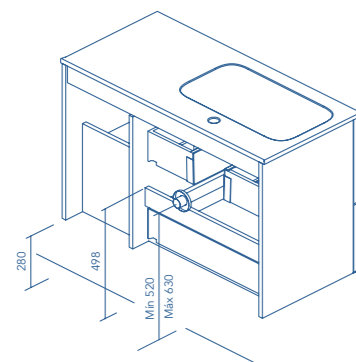
SANSA Fondo de tubería 7cm.
